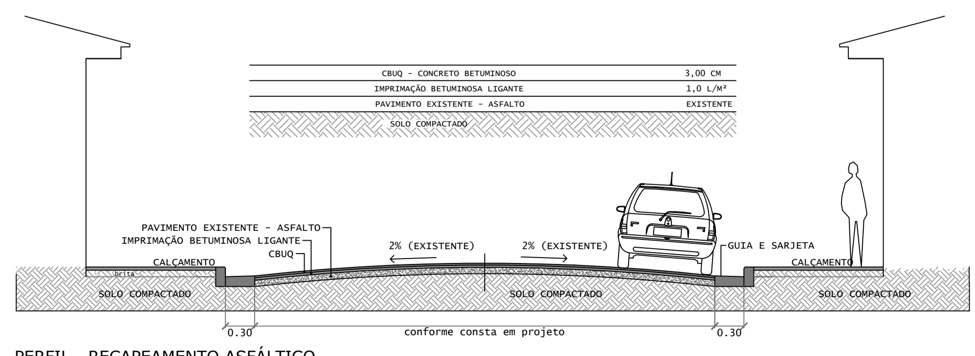
PERFIL - RECAPEAMENTO ASFÁLTICO SEM ESCALA
