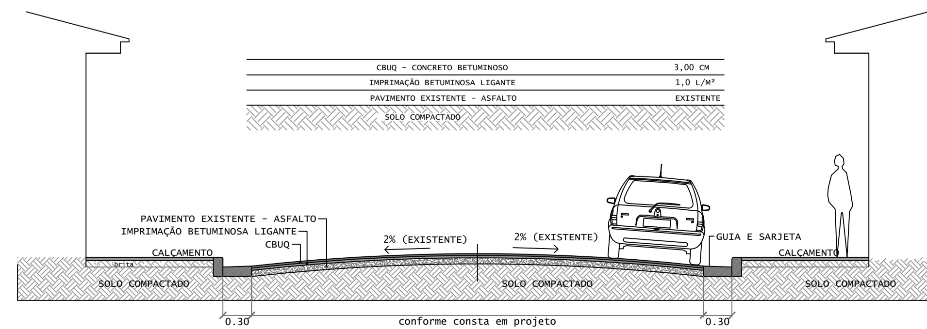
PERFIL - RECAPEAMENTO ASFÁLTICO SEM ESCALA
