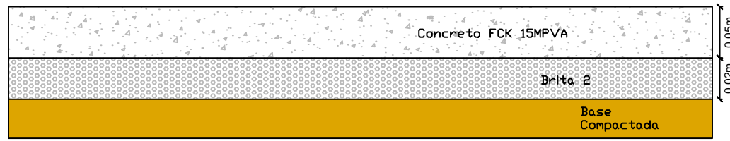
CORTE ESQ. (CALÇAMENTO) SEM ESCALA
