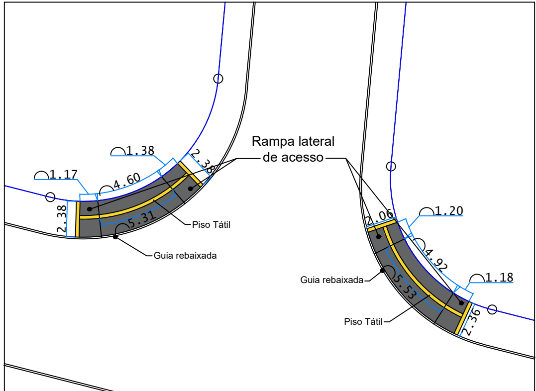
DETALHE 01 - RAMP ACESSÍVEL ESC. 1:250
