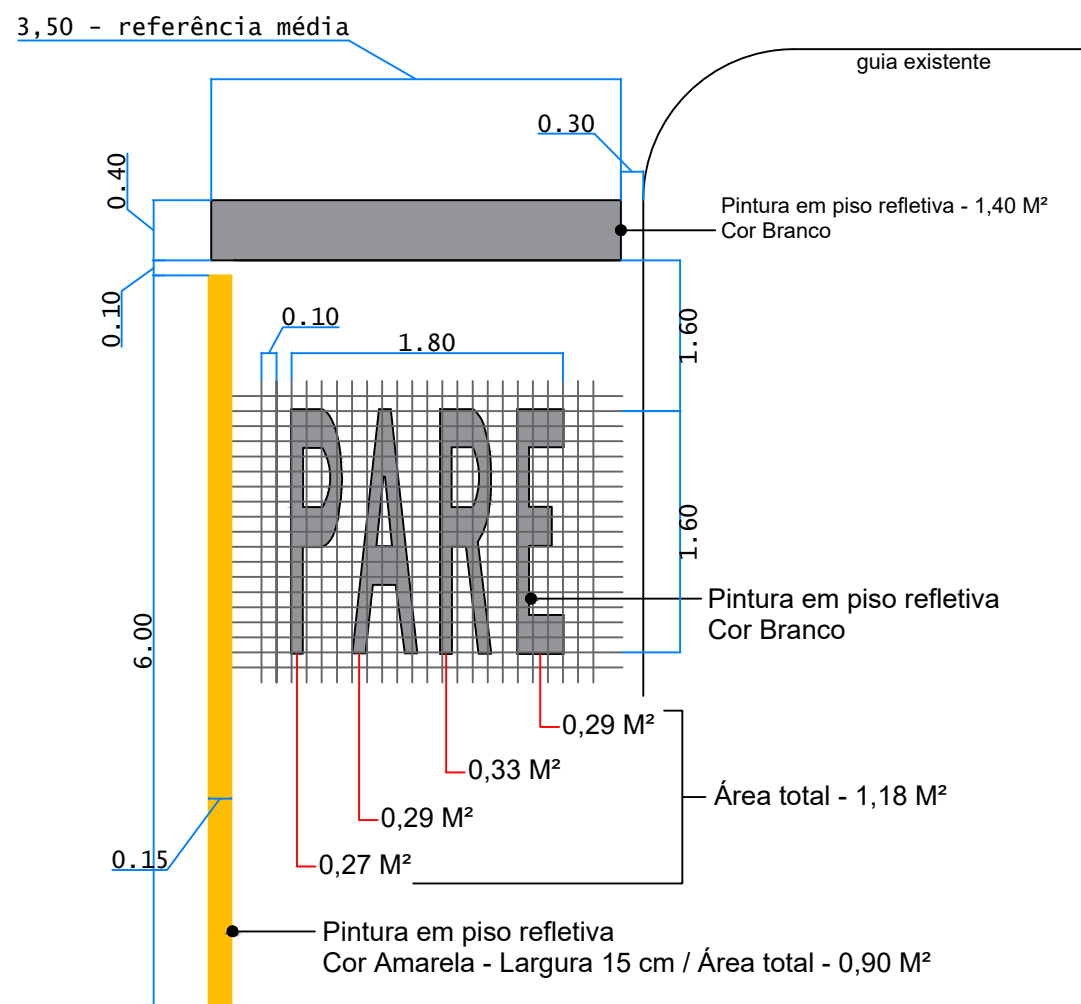
DETALHE SINALIZAÇÃO HORIZONTAL
