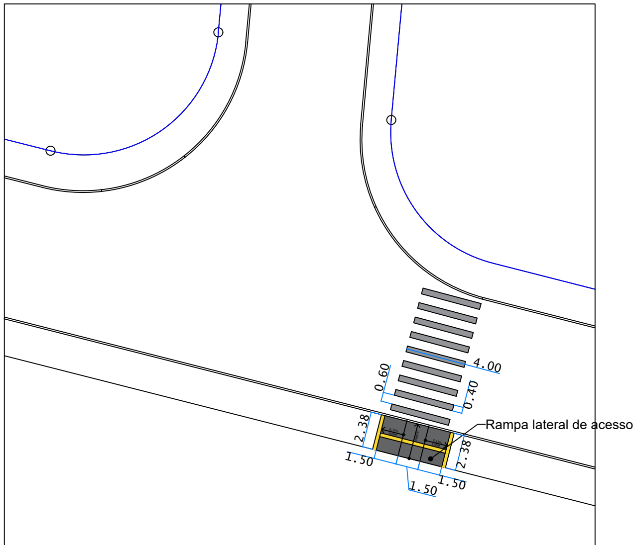
DETALHE 03 / FAIXA DE PEDESTRE + RAMPA ACESSÍVEL ESC. 1:250
