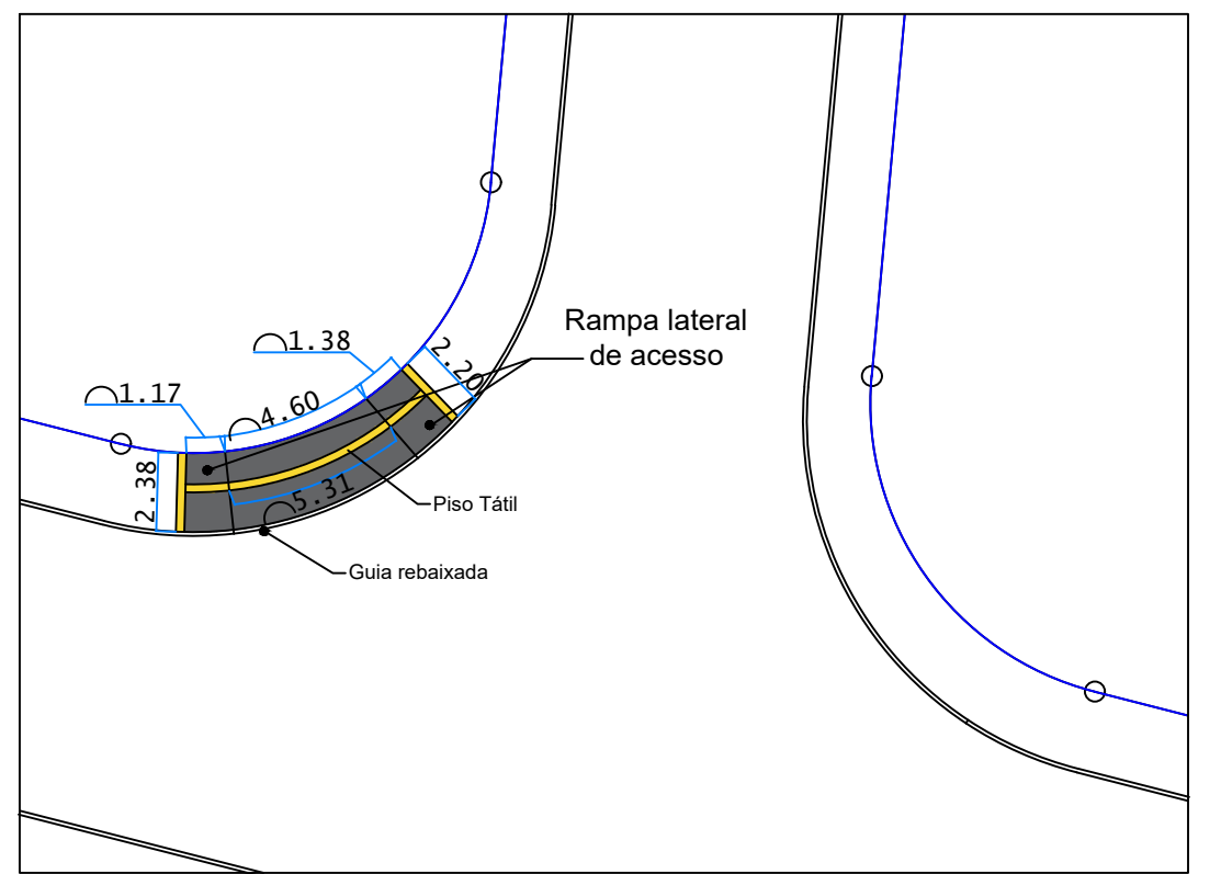
DETALHE 01 / RAMPA ACESSÍVEL ESC. 1:250
