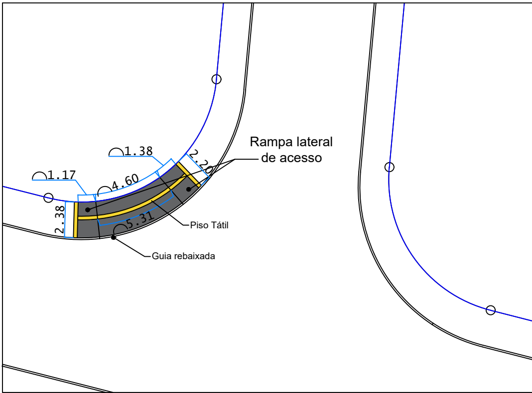
DETALHE 01 / RAMPA ACESSÍVEL ESC. 1:250
