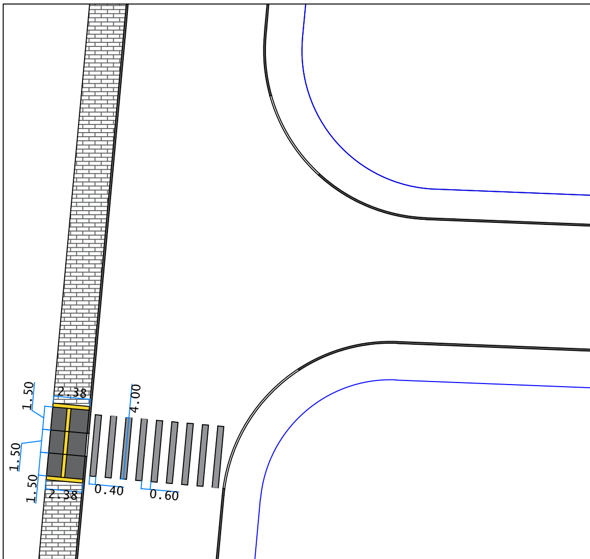
DETALHE 02 / FAIXA DE PEDESTRE + RAMPA ACESSÍVEL ESC. 1:250
